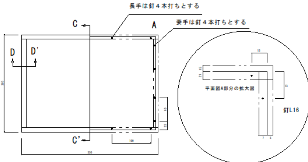
底板取付図S=1/1
