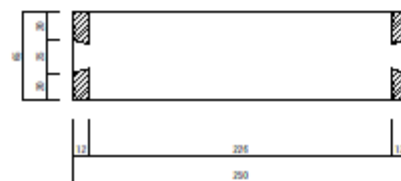
妻手側面図1/3
