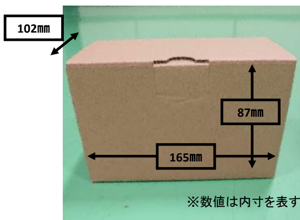
小箱完成図
