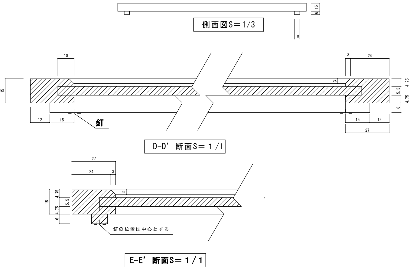
側面図 S=1/3
