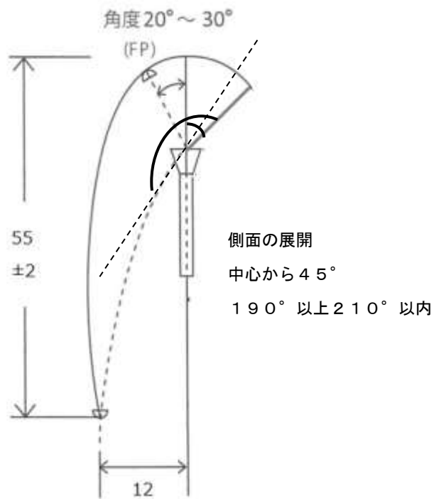
課題 2 （側面図）
