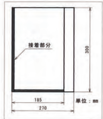
[図1 各部寸法]
