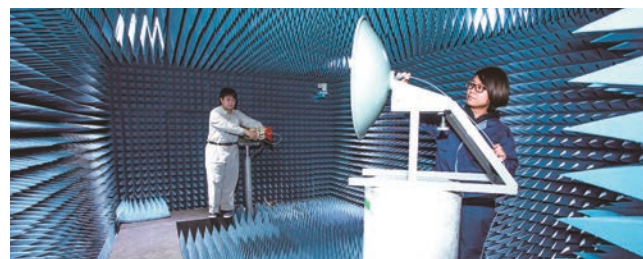
▲ 無線通信機器の特性測定
