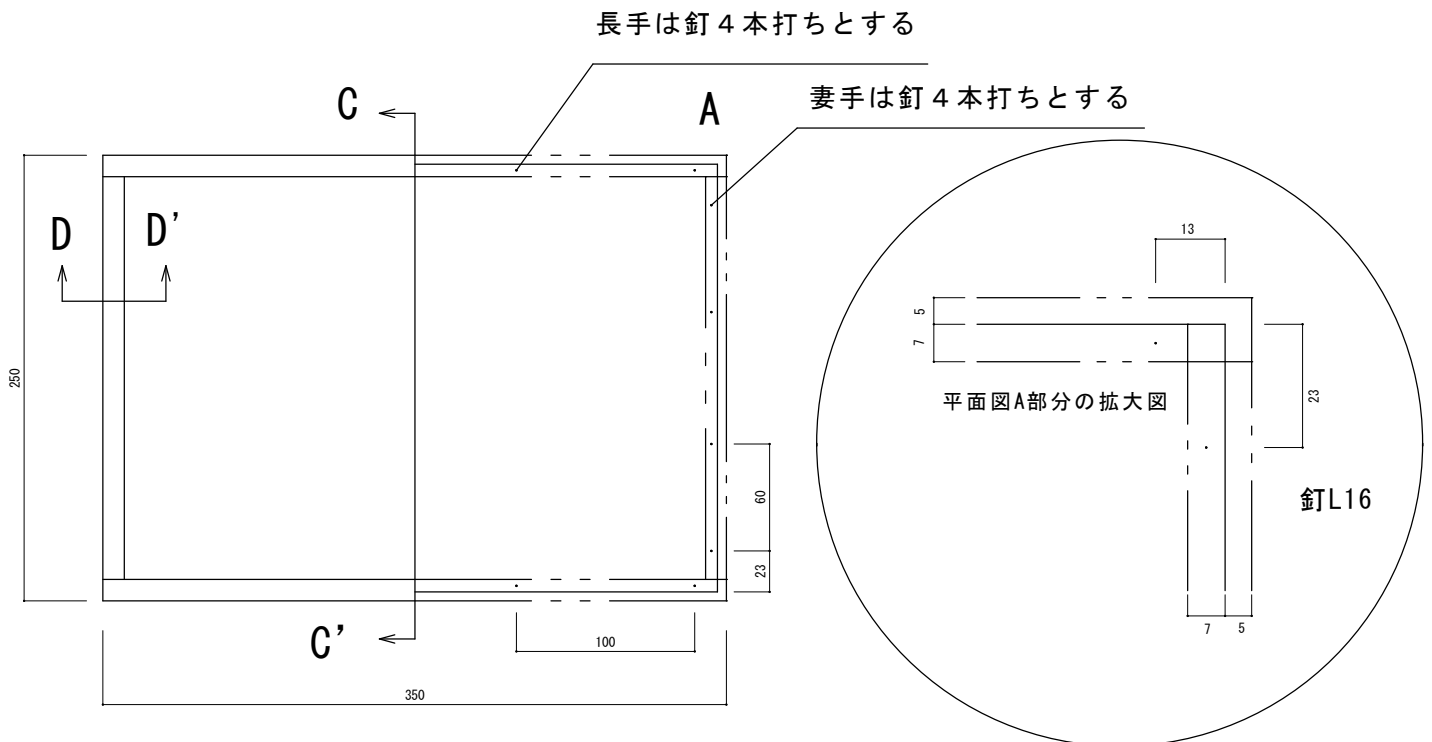
底板取付図 S=1/1
