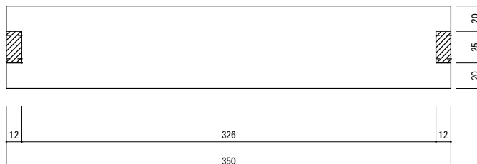
長手側面図 S=1/3
