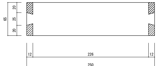
妻手側面図 1/3
