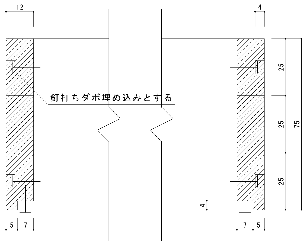
C-C' 断面図 S=1/1
