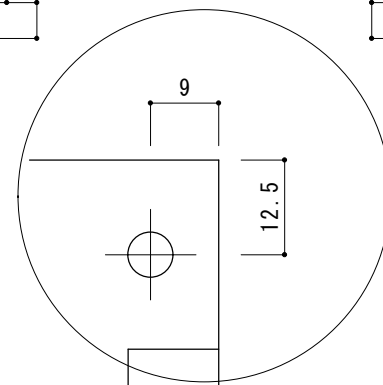
B部拡大図 S=1/1
