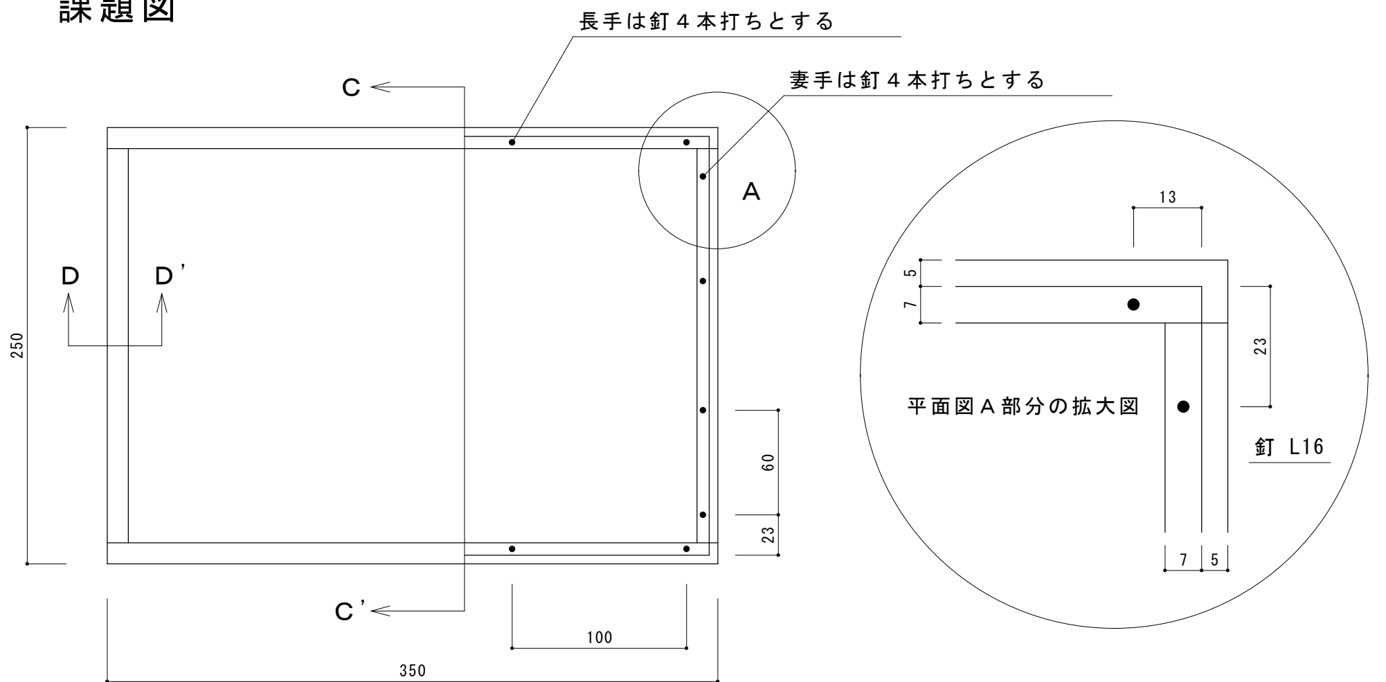
平面図 S=1/3
