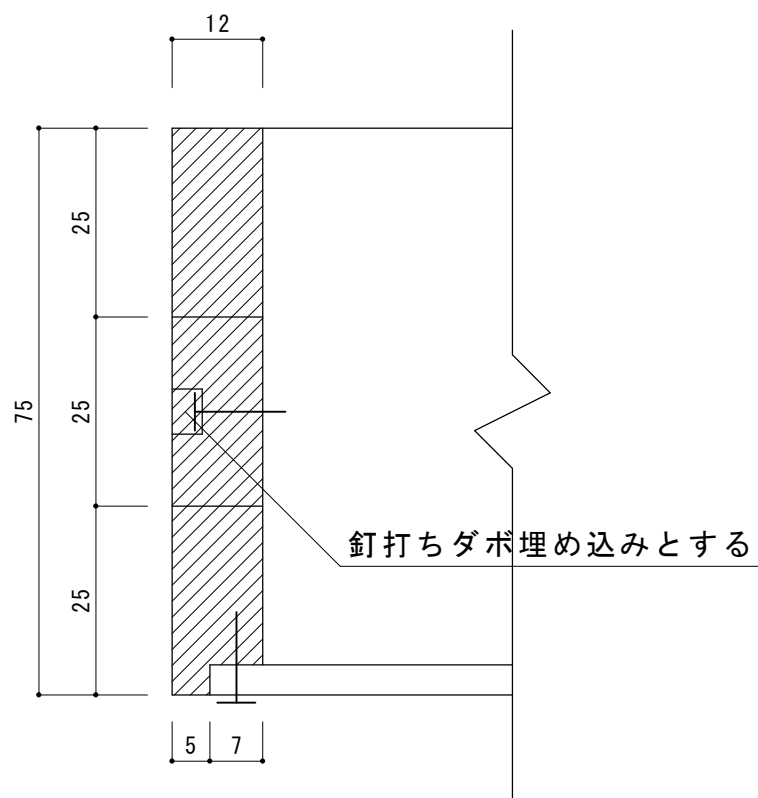
D-D' 断面図 S=1/1
