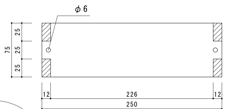
底板取付図 S=1/1
