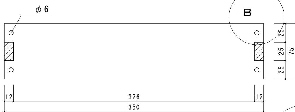
平面図 S=1/3
