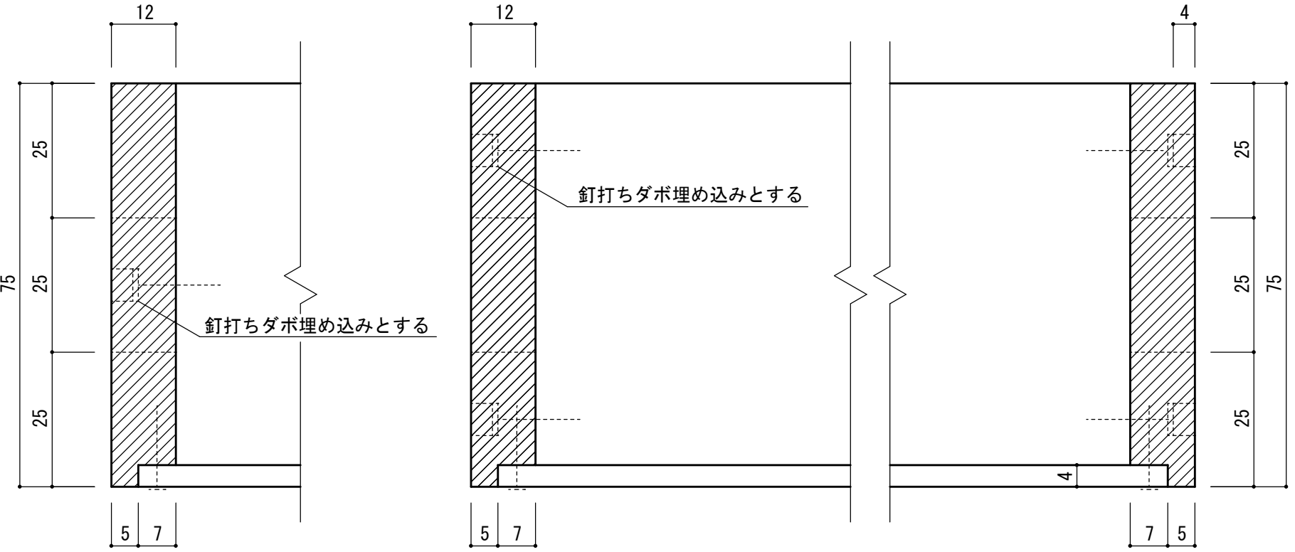
C-C' 断面図 S=1/1
