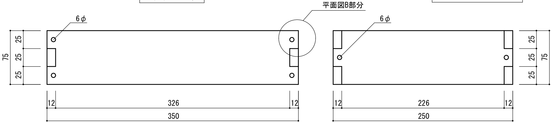
平面図 S=1/3
