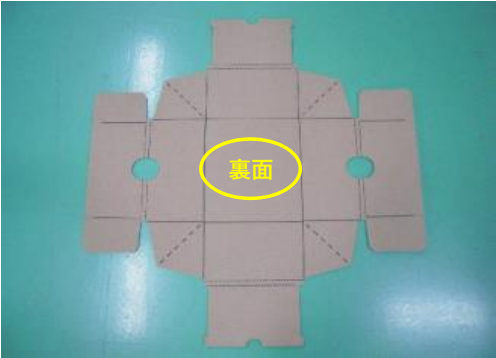
化粧箱蓋展開図
