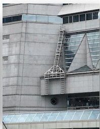
弊社設計エンジニア（講師）が設計製作したMMランドマークタワー自動窓面清掃装置
