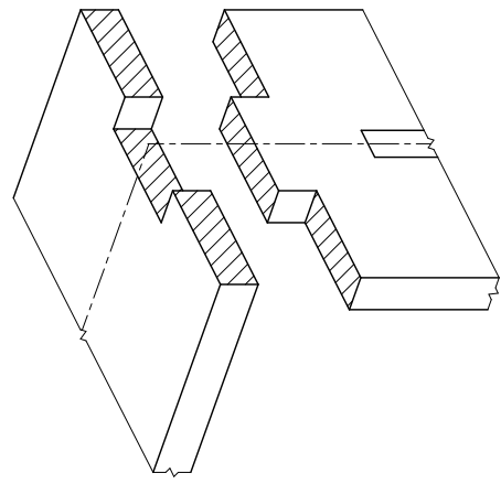
3枚組詳細図
