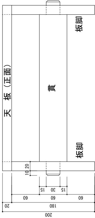
正面図
