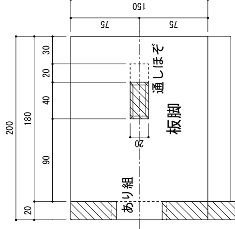
右側側面図
