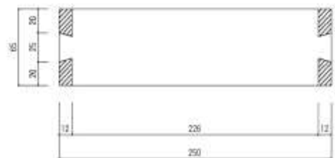
妻手側面図1/3
