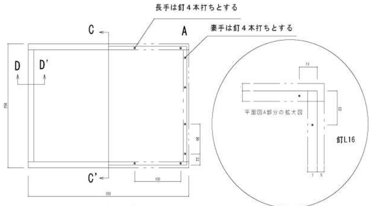
底板取付図S=1/1
