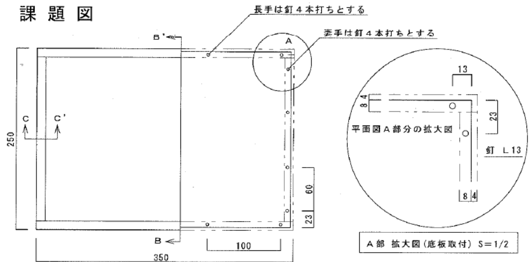
平面図 S=1/4
