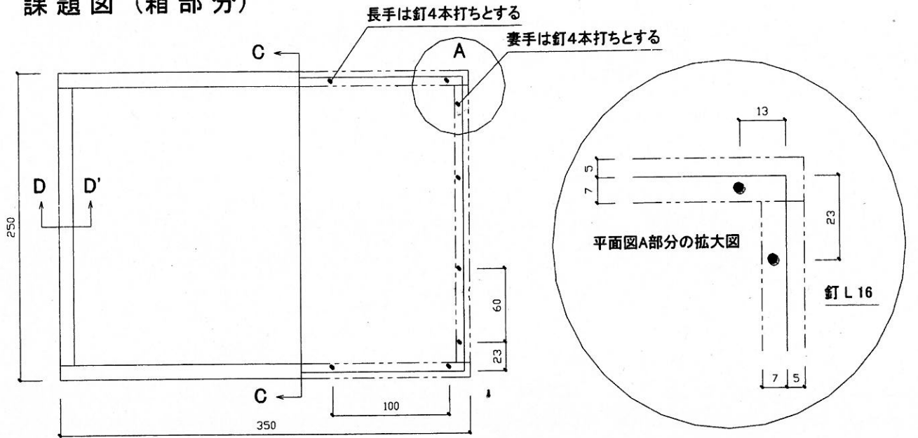
平面図 S=1/3
