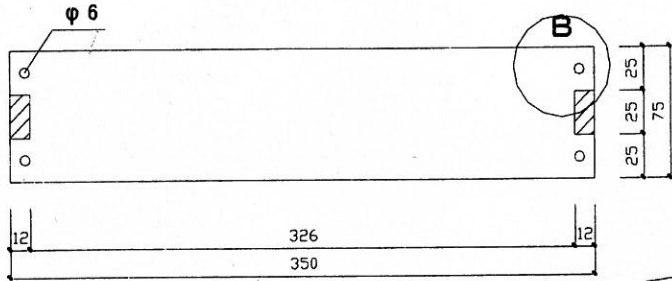
長手側面図 S=1/3
