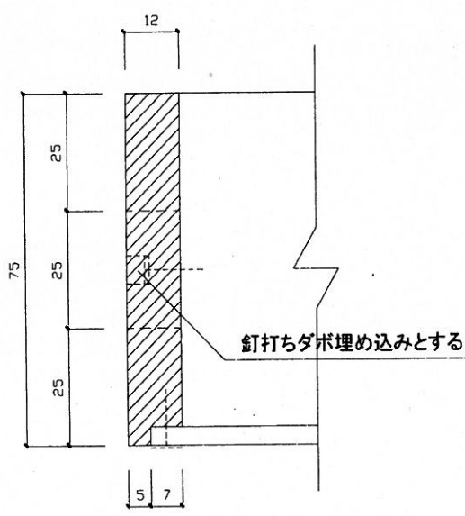
D-D' 断面図 S=1/1
