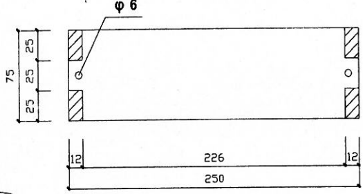
妻手側面図 S=1/3
