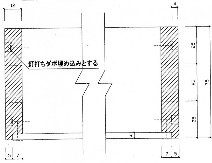
C-C' 断面図 S=1/1
