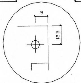
B部 拡大図 S=1/1
