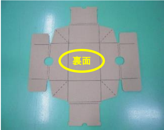
け しょう ぼこ ふた てん かい ず 化粧箱蓋展開図
