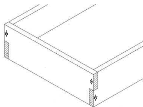
二枚組接ぎ納まり図S=1/3
