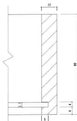
底板納まり図S=1/1
